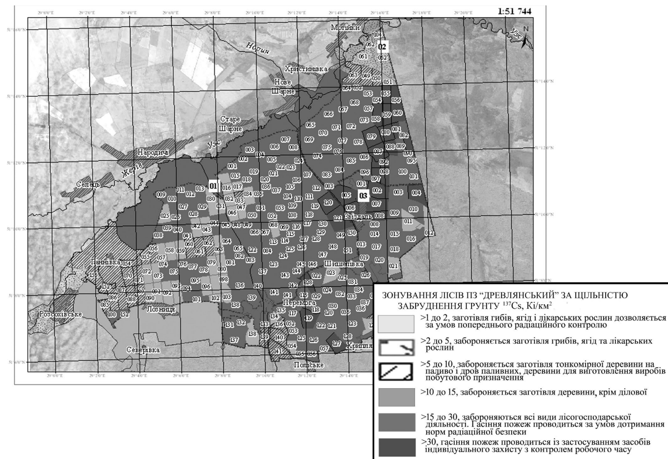
Рис. 2. Зонування території лісництва (01 — Народицького; 02 — Заліського; 03 — Кліщівського) у ПЗ «Древлянский» за щільністю забруднення ґрунту ^{137}\text{Cs} станом на 2023 р. (див. кольоровий рисунок на сайті журналу)
