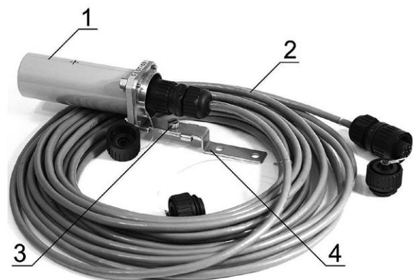
Рис. 1. Зовнішній вигляд БД БДБГ-09 (1) зі з'єднувальним кабелем (2), фіксатором (3) і кронштейном кріплення до стіни (4)
